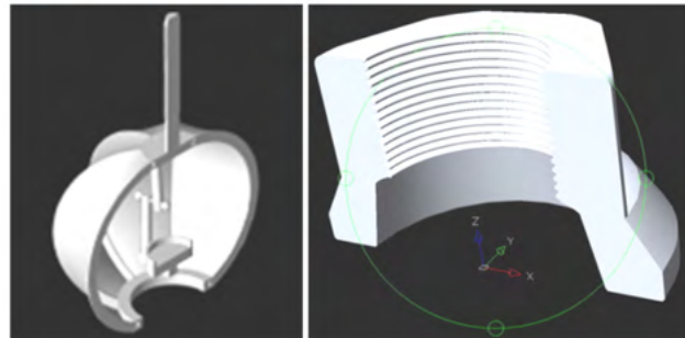
거푸집연결구 (30-0994347)
