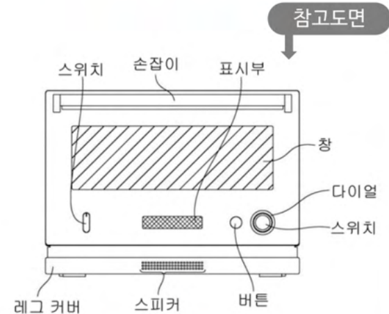
전자레인지 (30-0979613)
