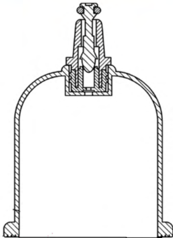
〈두께를 표현한 단면도〉
